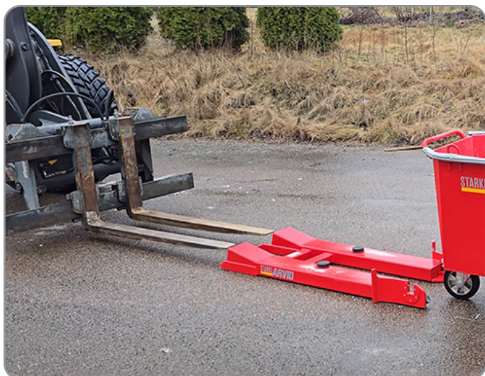
Affaldsvognstømmere løftes nemt op direkte med gaffeltruckens gaffer.
