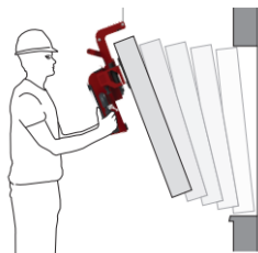
Fönstret lyfts med den elektriska fönsterlyften till önskad höjd och lutas in mot fönsteröppningen.
