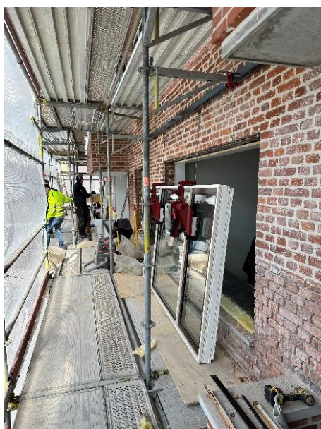
Den patenterade pivot-armen gör att fönstret placeras i fönsteröppningen med nederdelen först.
